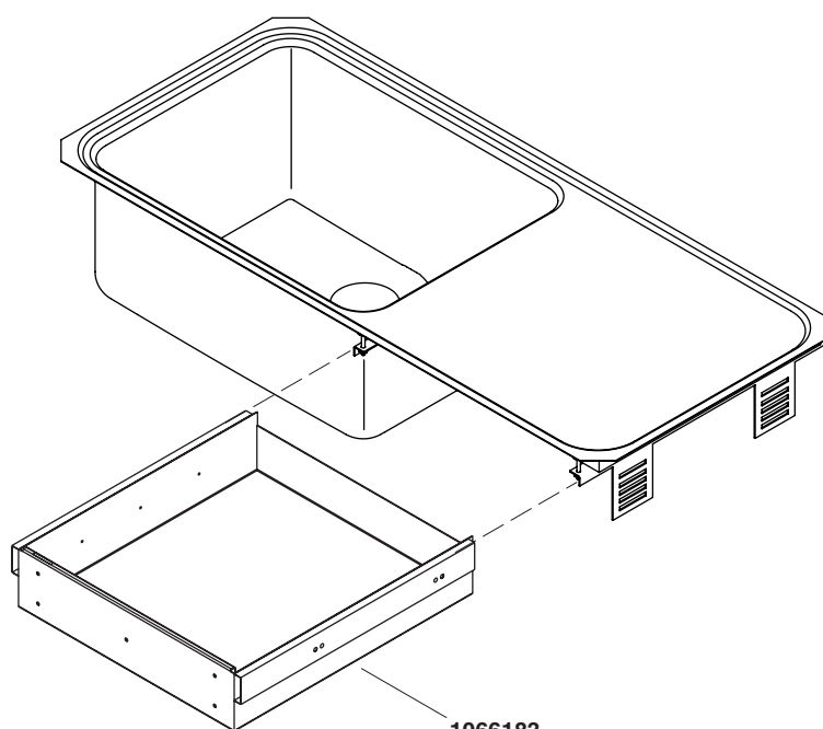
1066183 Montaje del cajón
