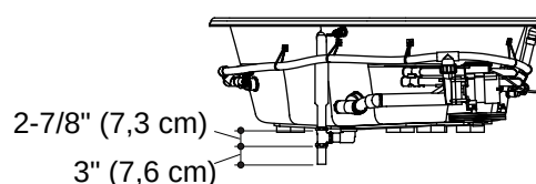
Détail de la découpe du style rebord intérieur
