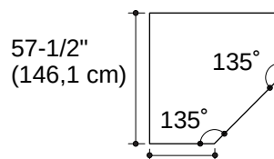
Détail de la découpe du style rebord intérieur
