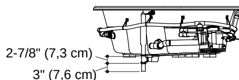
Detalle de la abertura de los modelos con borde empotrado
