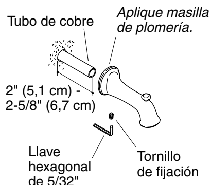
Surtidor de montaje deslizante
