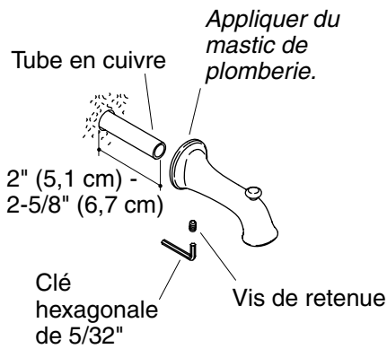
Bec à montage tournant
