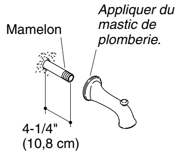
Bec fileté
