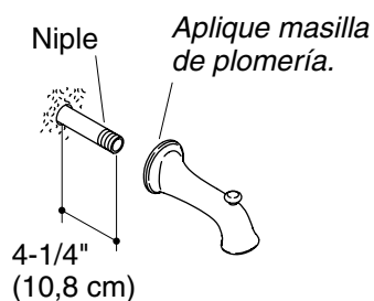
Surtidor roscado
