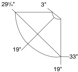
1703-90 Corner 90° Hang Table
