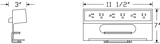
6 simplex receptacles
