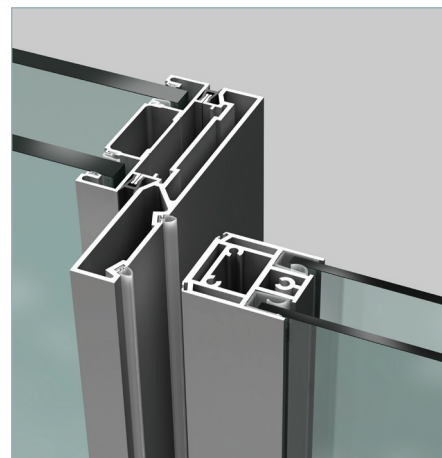
LOCKING JAMB
