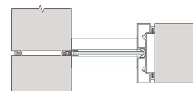
FILLER FIN
