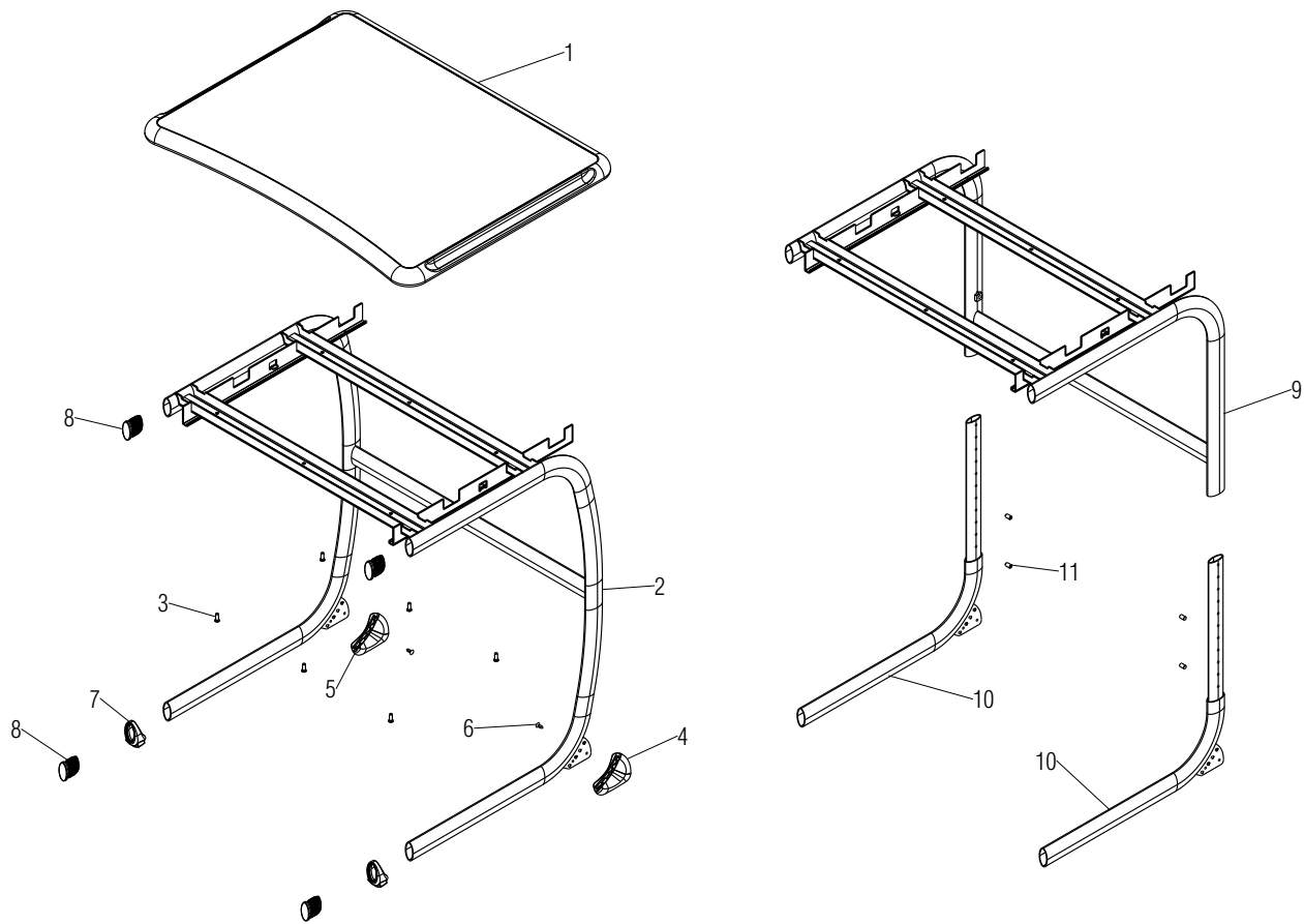
S, M, L & XL Height Desk
