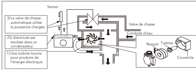
fig. 1 Générateur Hydropowered
