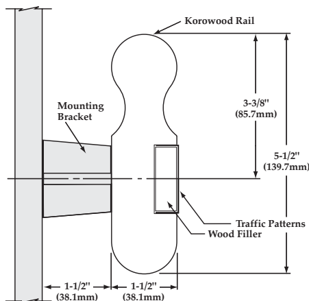
HW20-TP
