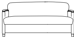
734-3, Sofa W=70½", D=27½", H=32½", SH=18", AH=23¾"
