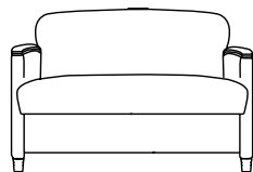
734-2, Settee W=49", D=27½", H=32½", SH=18", AH=23¾"
