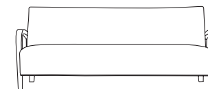
736-3, Sofa W=72", D=29½", H=32", SH=18½", AH=23"
