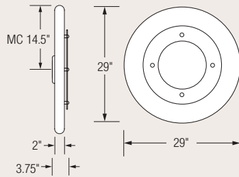
OIW1010 ADA
