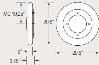
OIW1000 ADA
