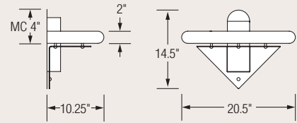
OIW1002
