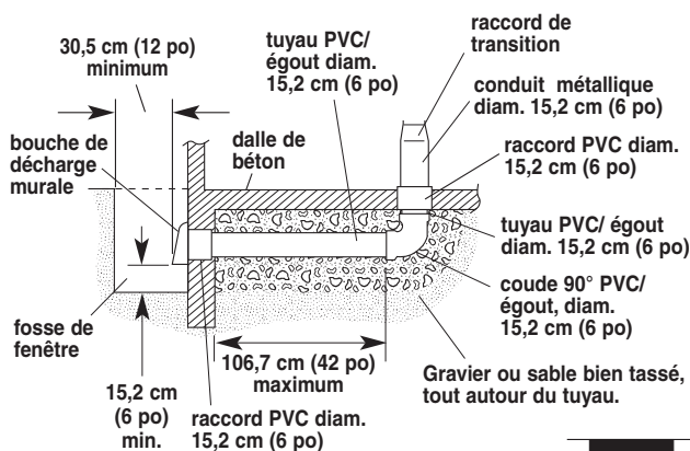
option - circuit d'évacuation installé sous une dalle de béton, dans une fosse de fenêtre.
